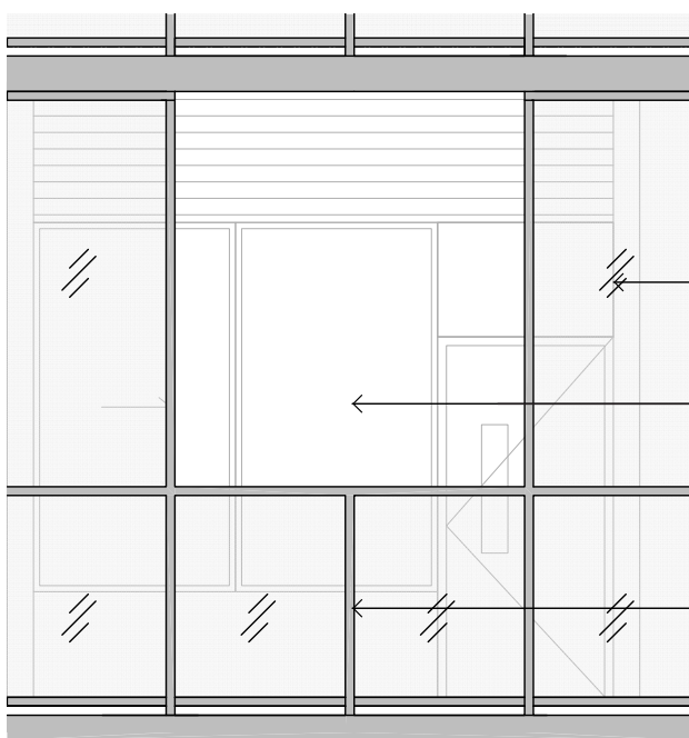
Elevation - glazing
